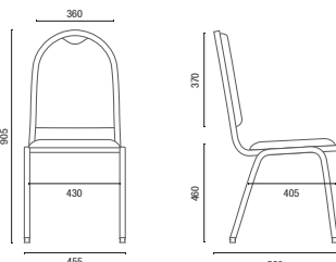
1002 Empilhavel
